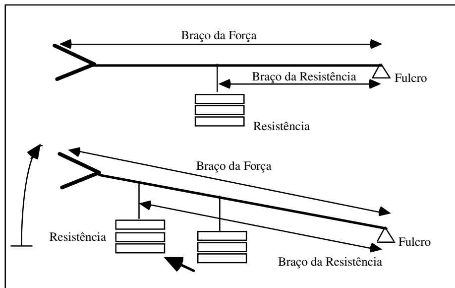
Figura 17 Alteração do braço da resistência numa máquina de resistência progressiva
